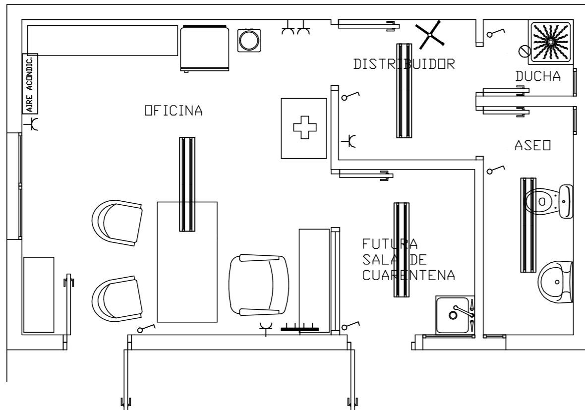
INSTALACION ELECTRICA
