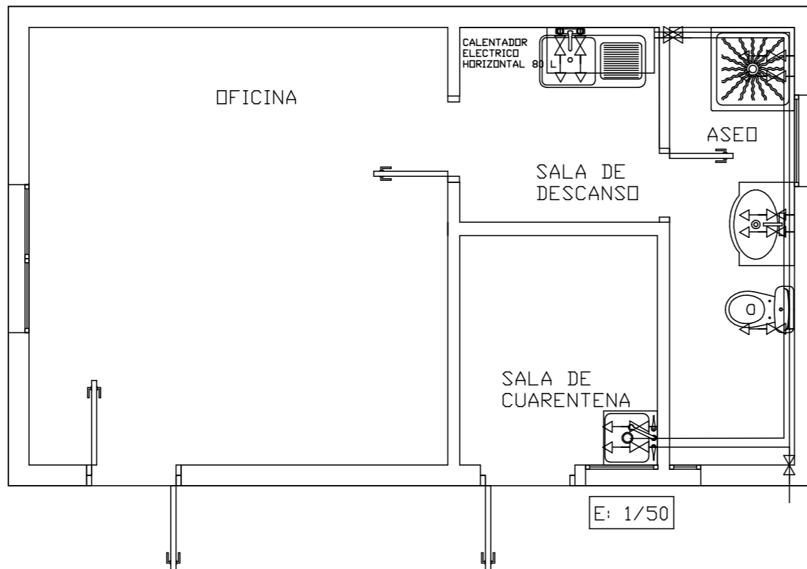
FONTANERIA
