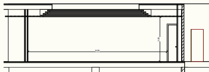
Secció transversal 1
